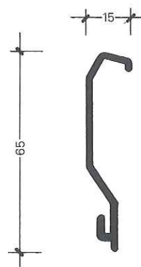
Wandaansluitingsprofiel
